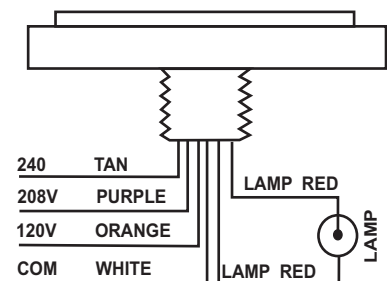
120/208/240 VOLT CONNECTION
