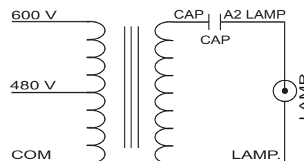
480/600 VOLT CONNECTION
